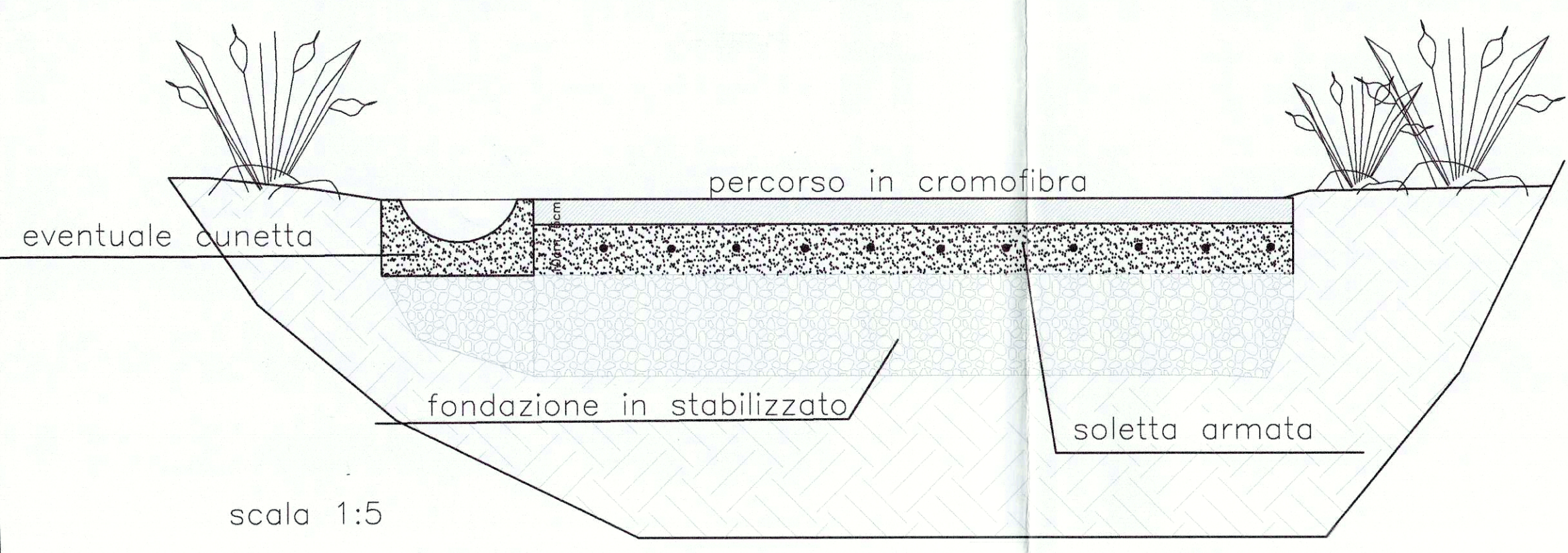
PARTICOLARI TECNICI (sezione dei percorsi e delle rampe di scale)
