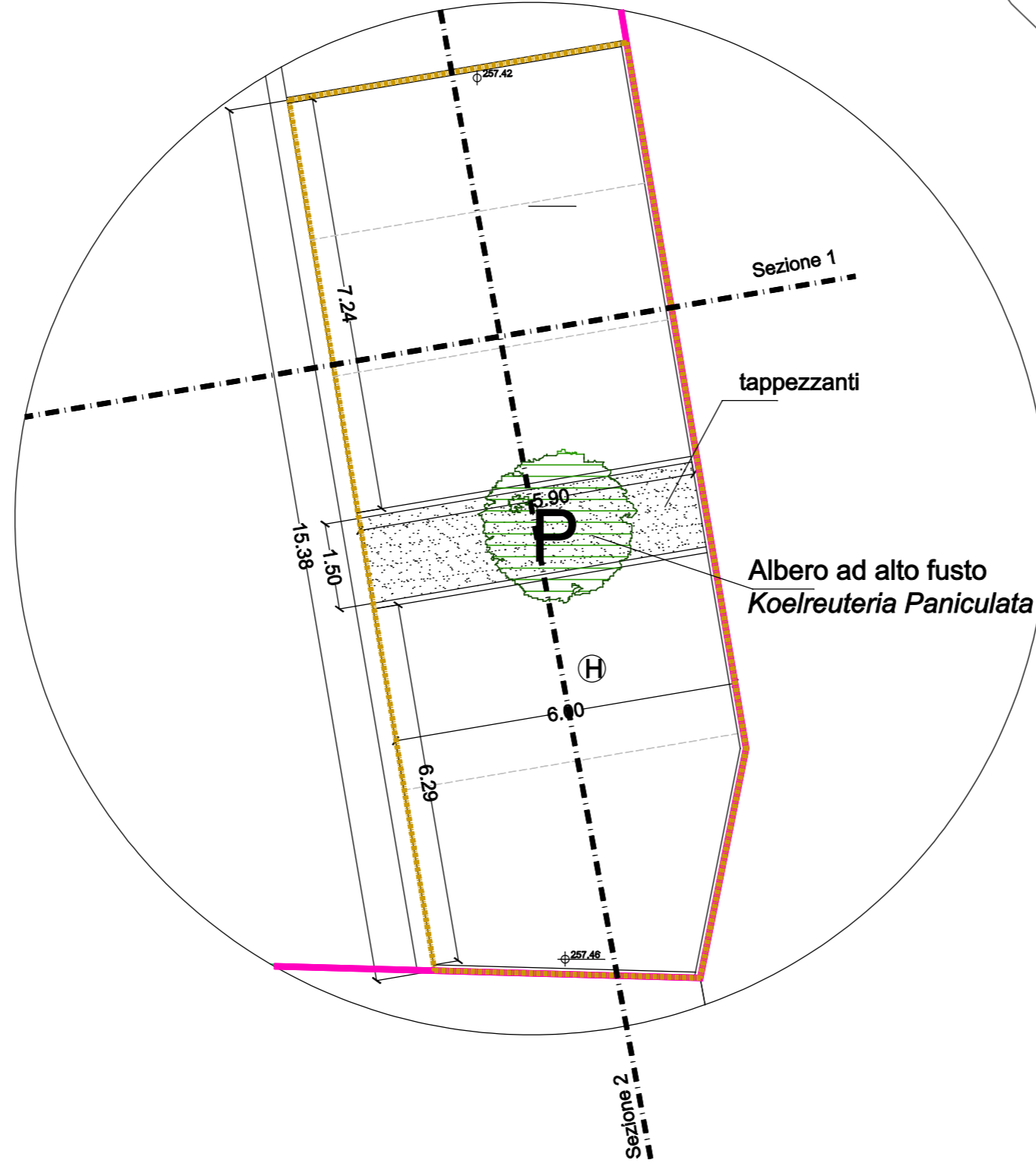
Particolare 1 Scala 1:100
