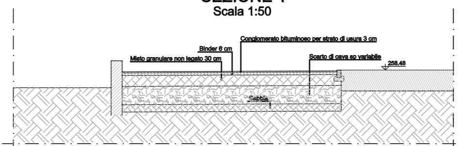
SEZIONE 1 Scala 1:50
