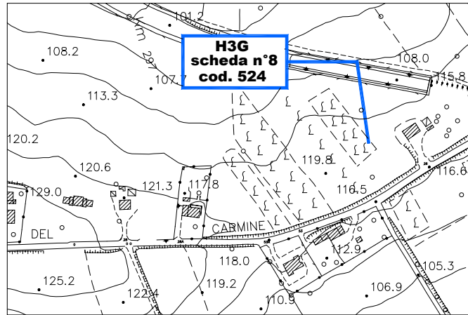
Stralcio aerofotogrammetrico scala 1:5000 Tav. 293024V
