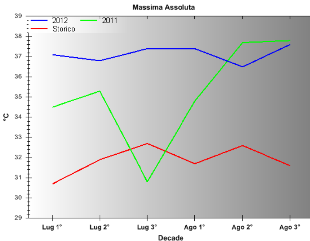
Figura 2 – Andamento della temperatura massima assoluta di luglio-agosto
