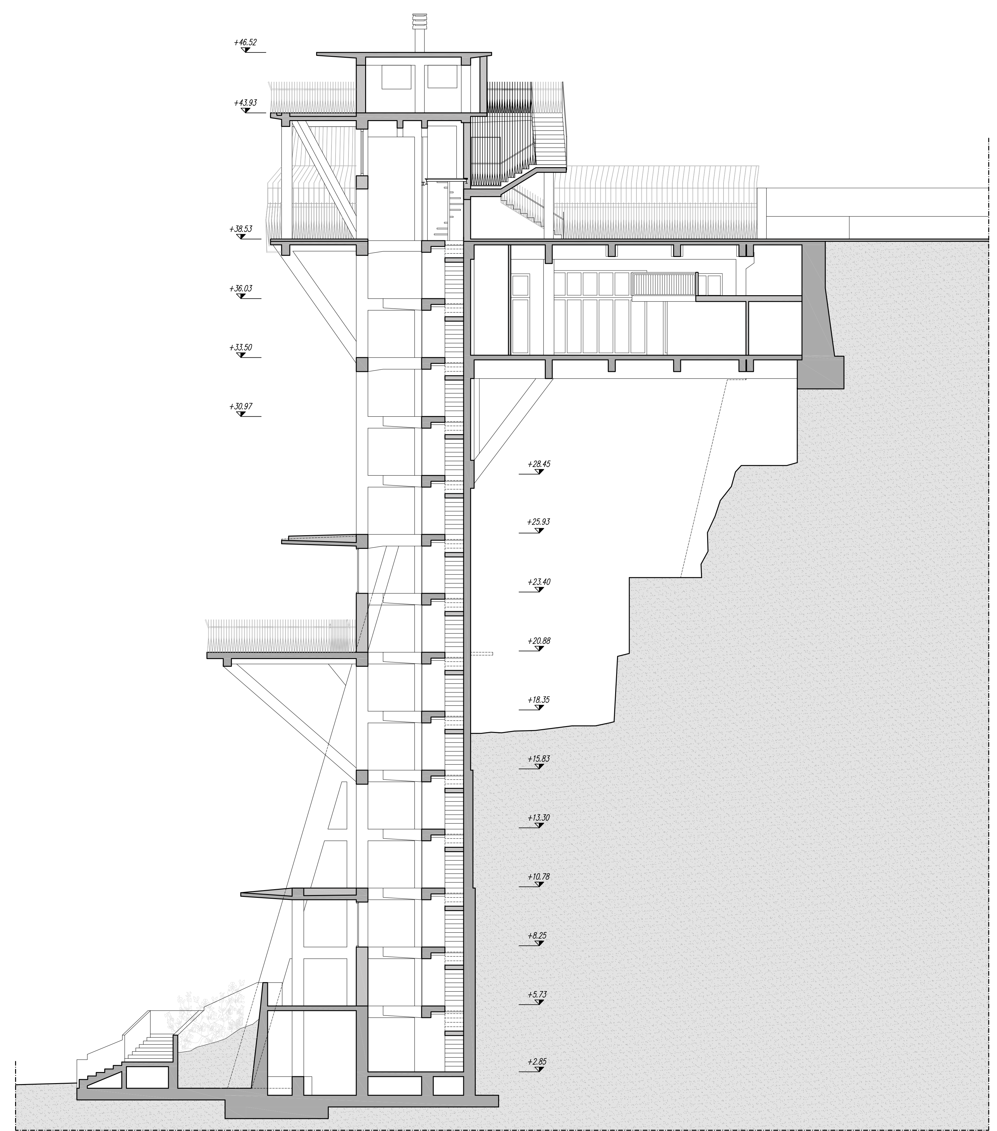
SEZIONE AA
