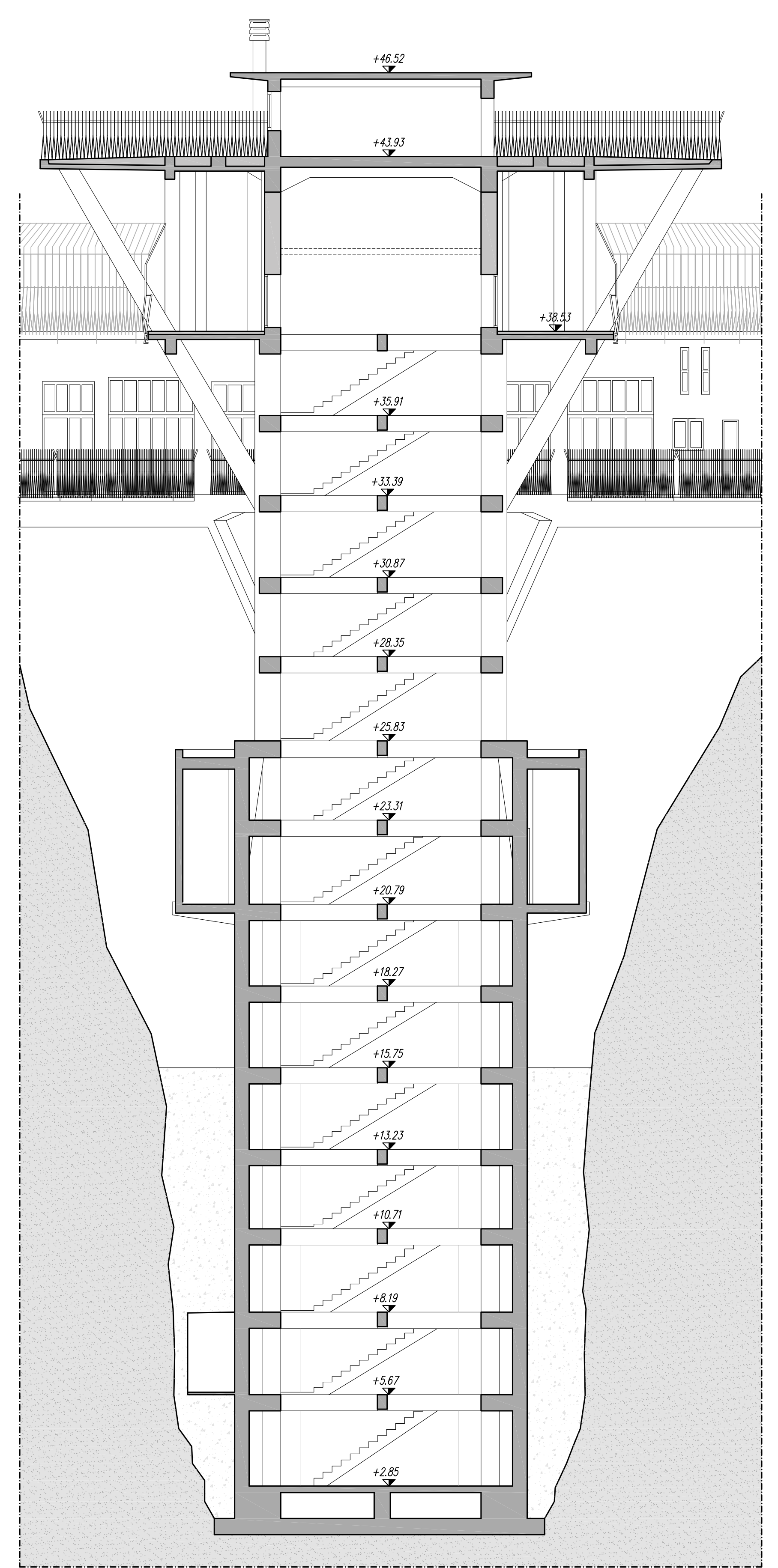
SEZIONE CC
