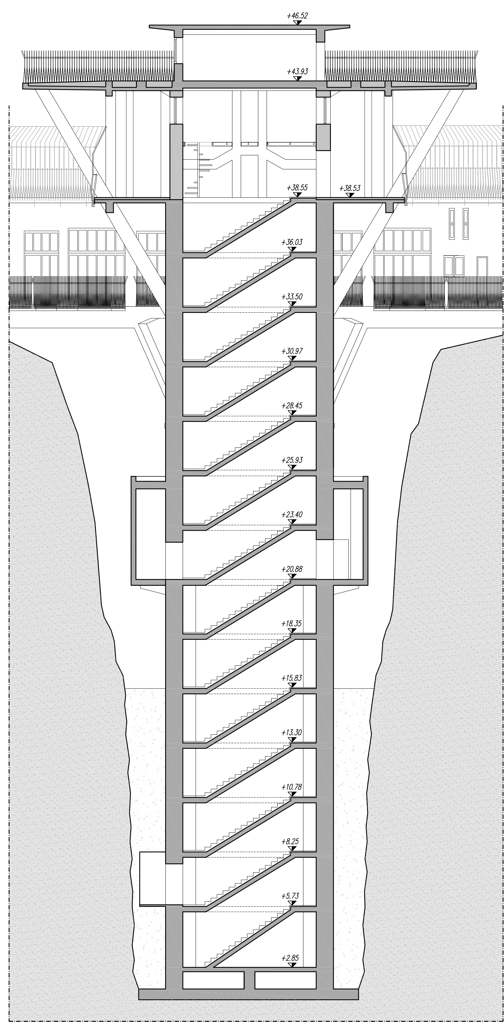
SEZIONE BB
