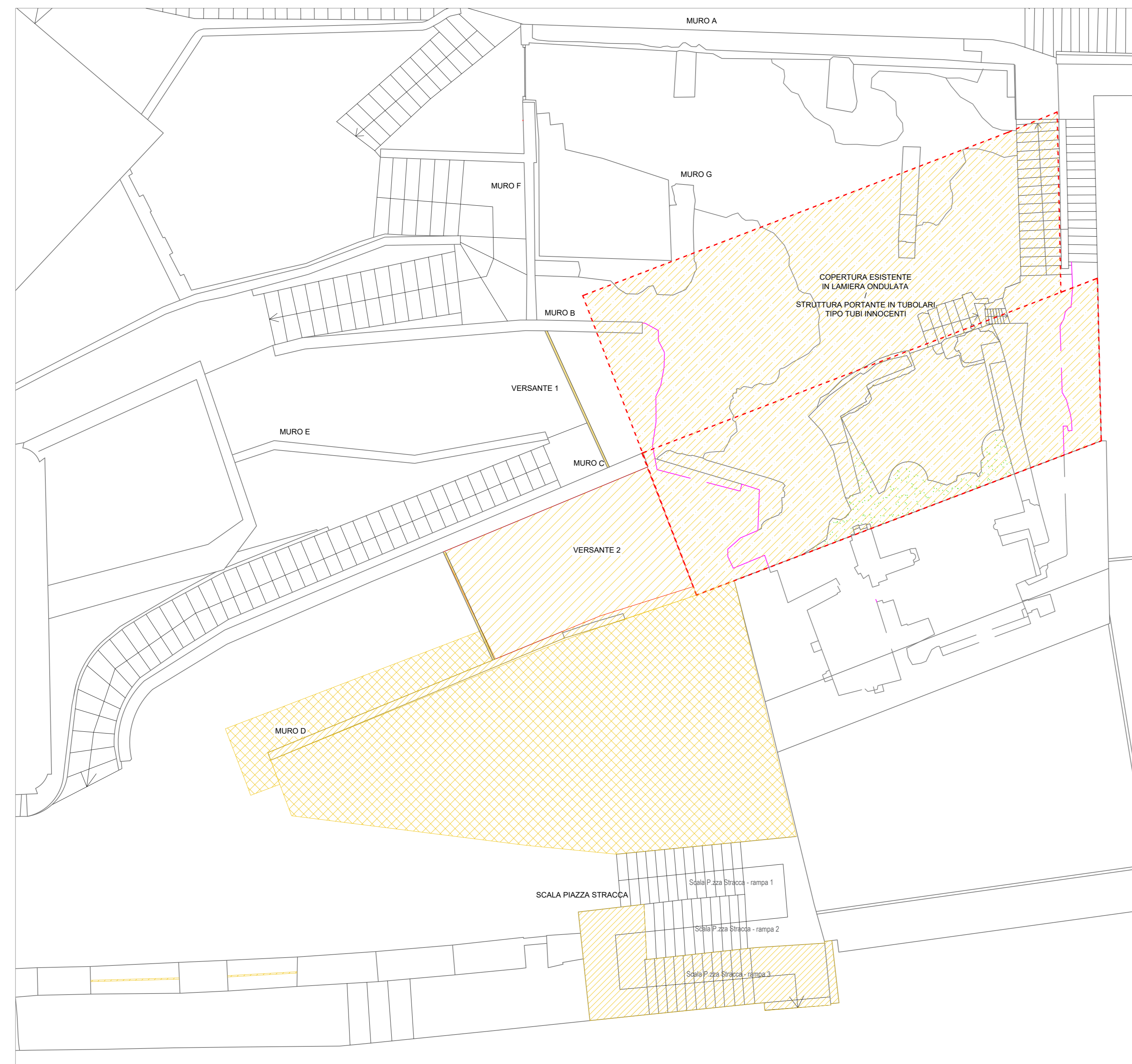
1 Pianta +34 - Demolizioni Scala 1:100
