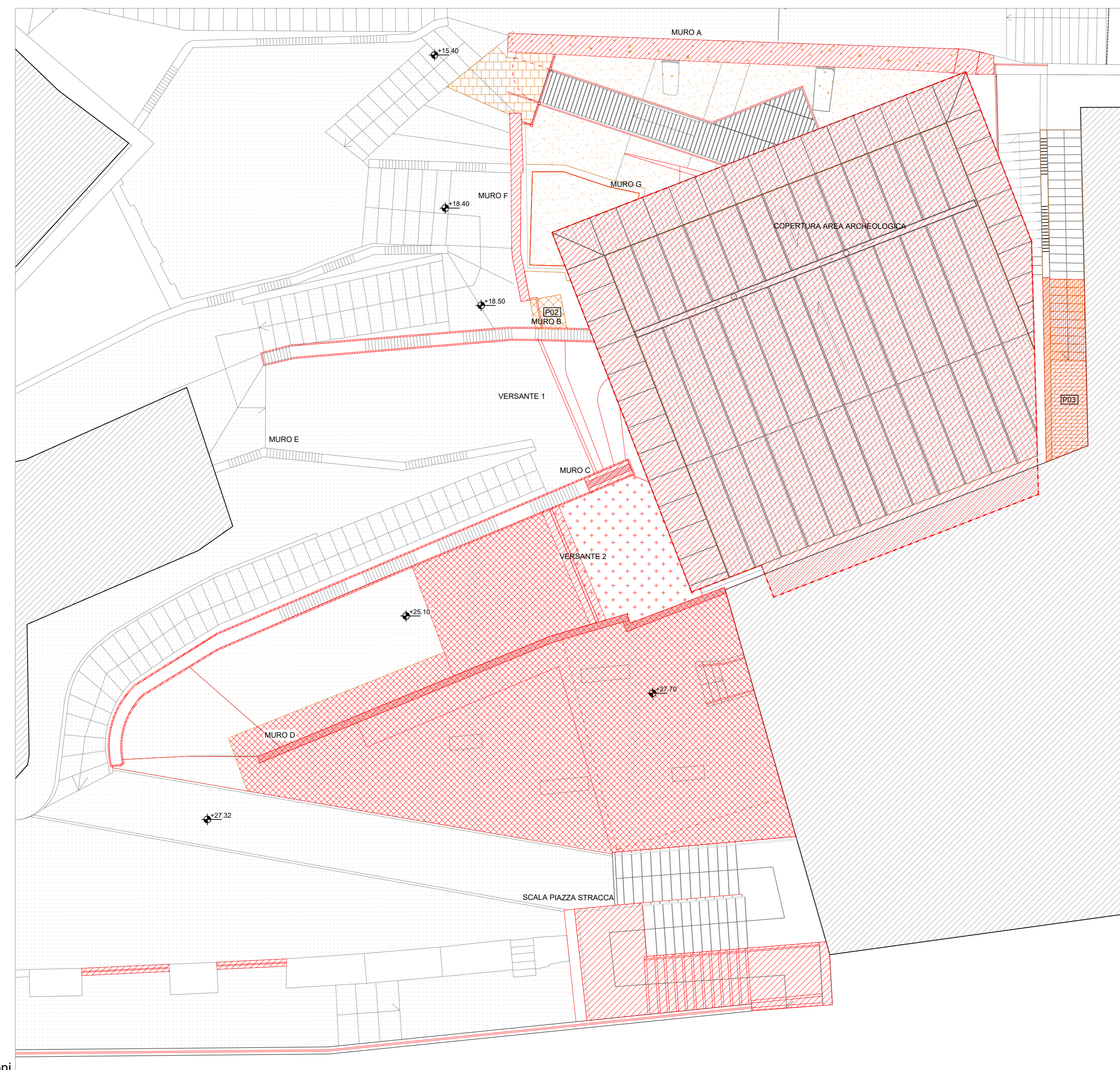
1 Pianta +34 - Demolizioni Scala 1:100
