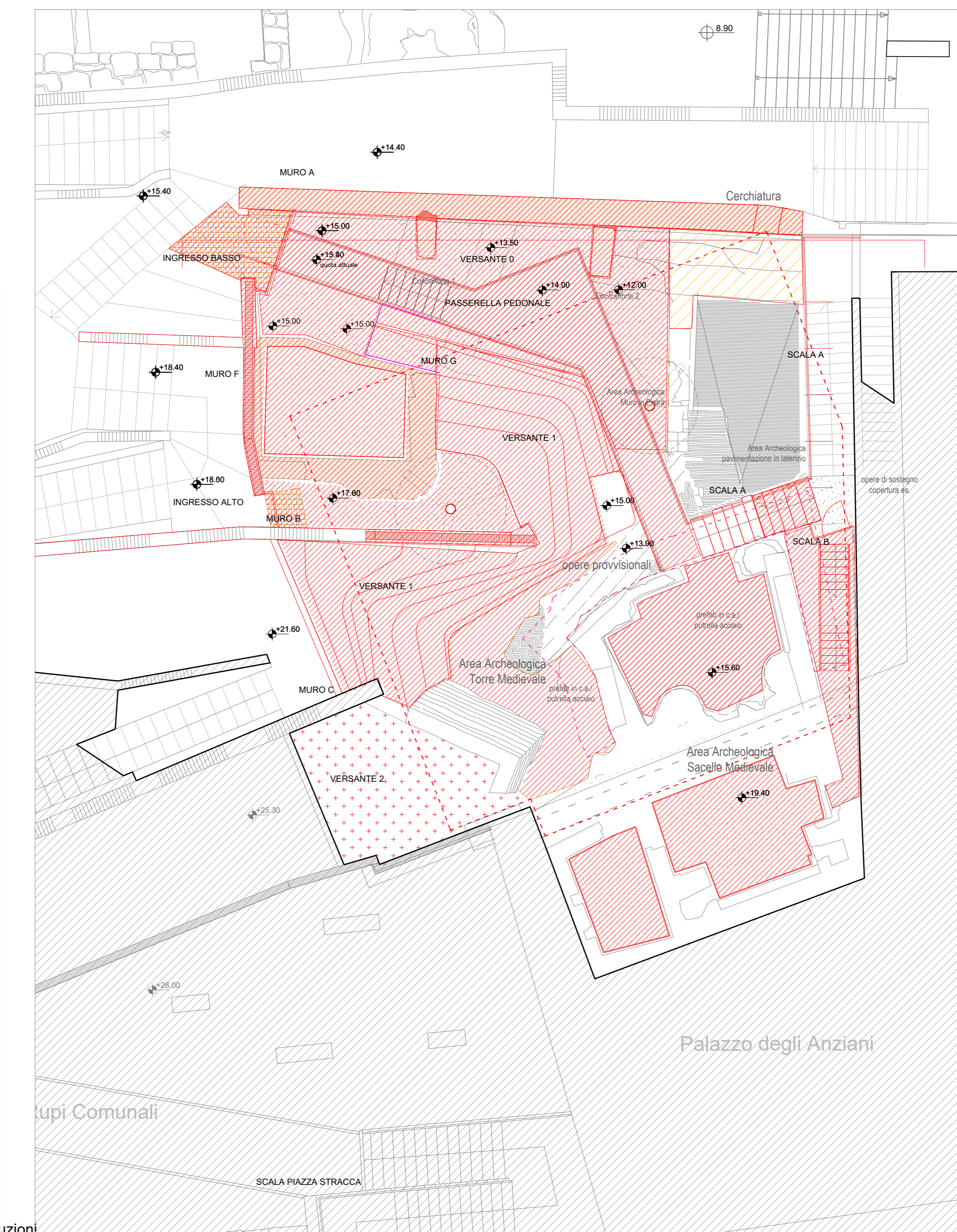
2 Pianta +23 - Demolizioni Scala 1:100
