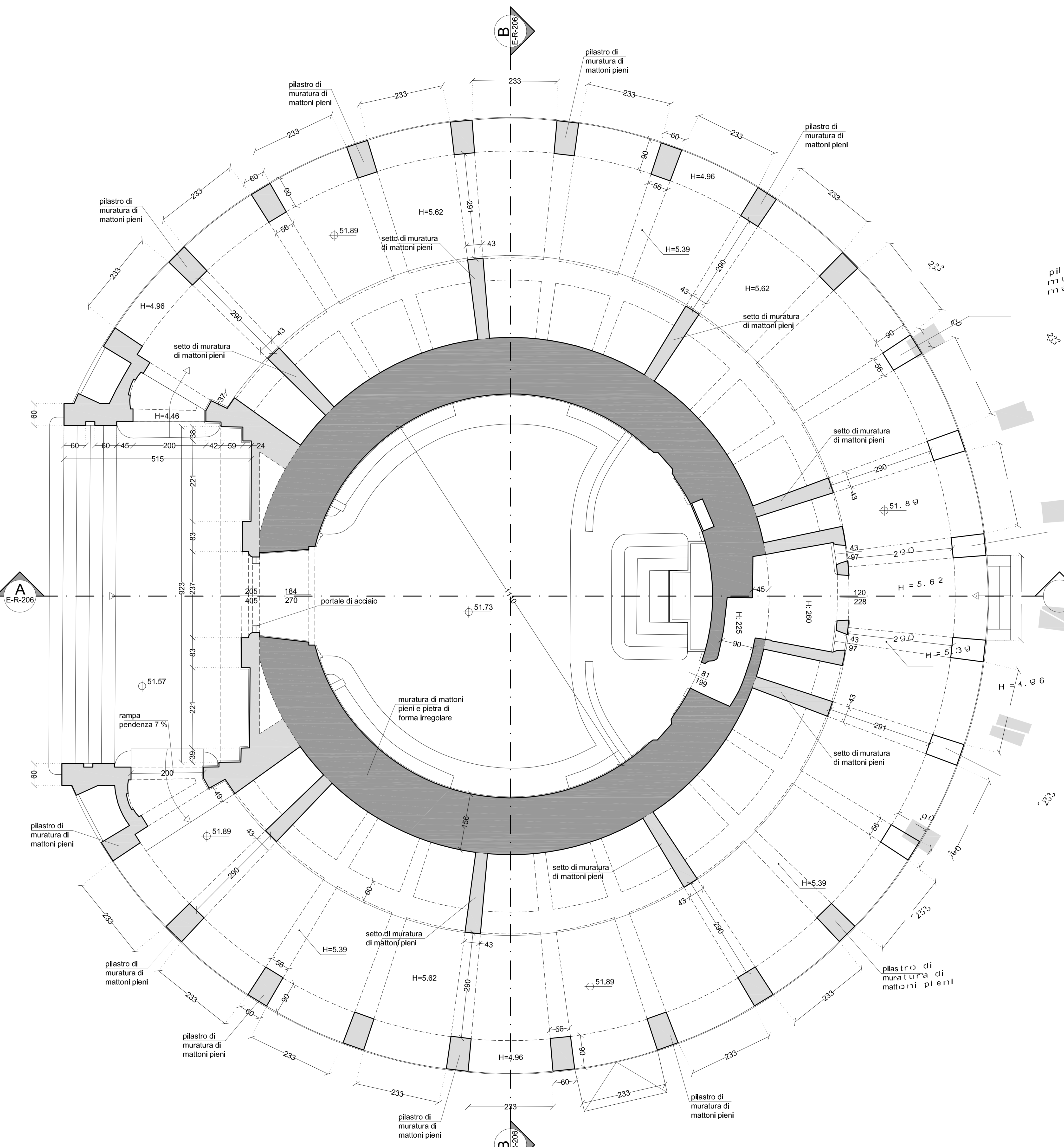
PIANTA QUOTA TERRENO
