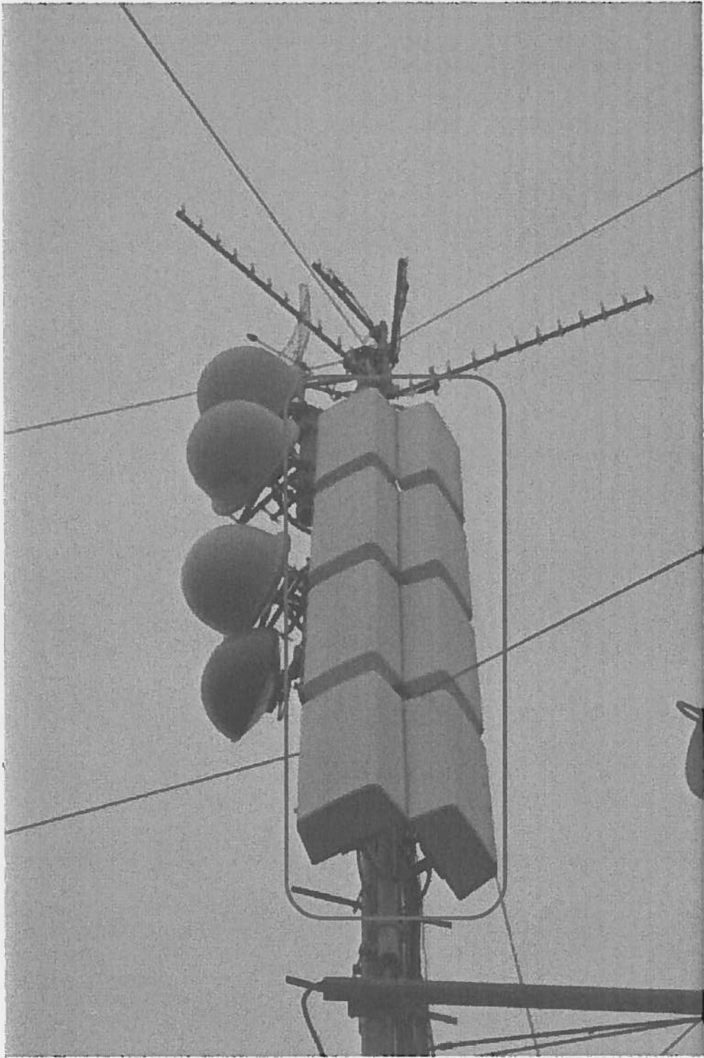
Dettaglio fotografico del sistema radiante
