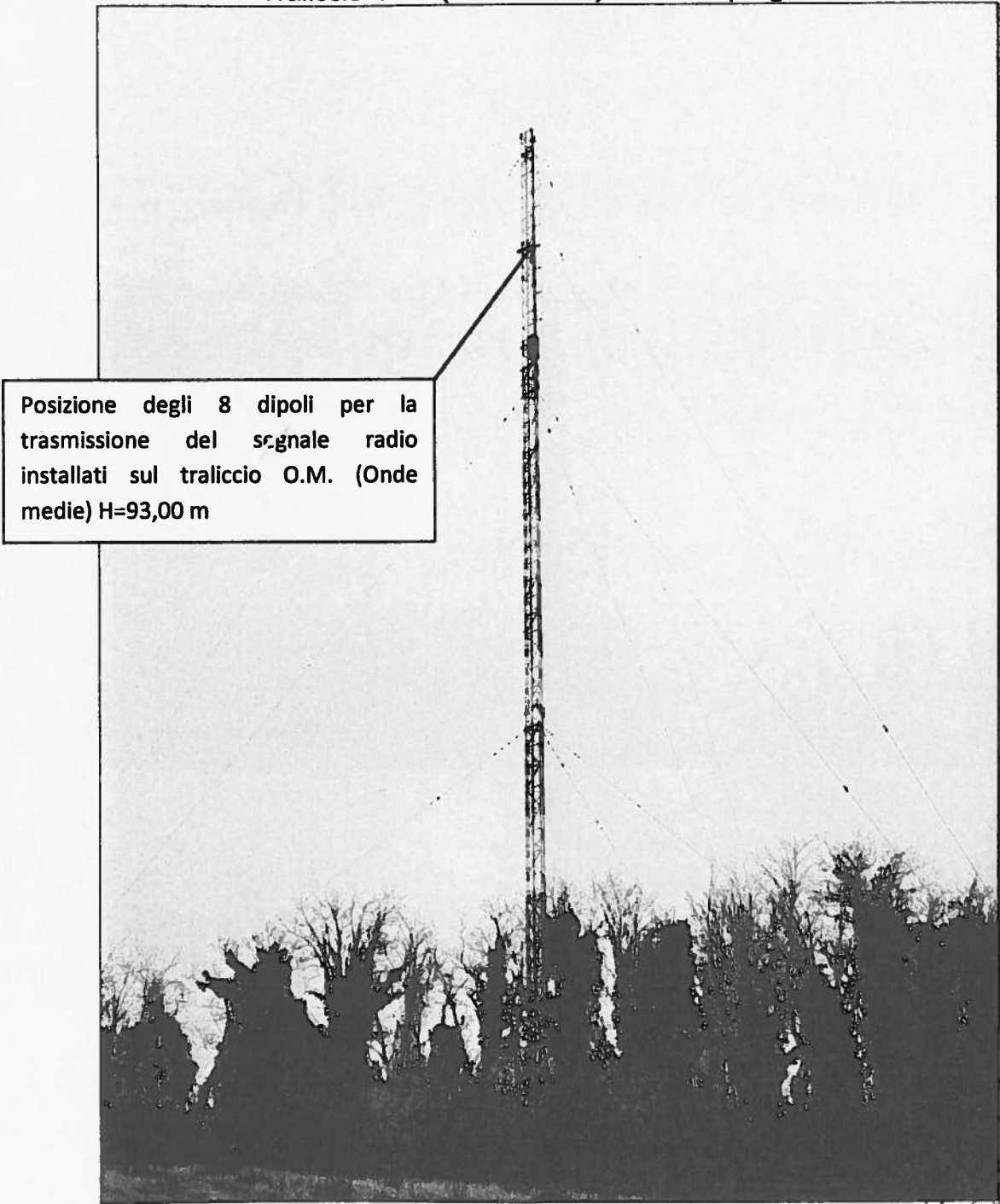
FOTO 7 Traliccio O.M. (onde medie) - stato di progetto
