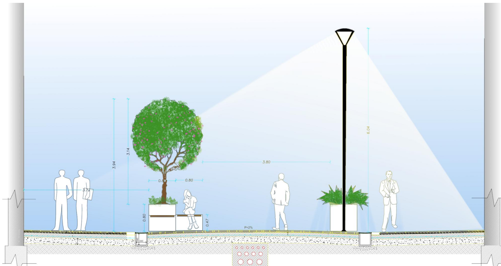
SEZIONE STRADALE TIPO
